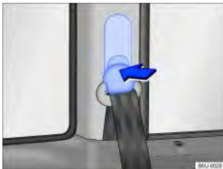
Fig. 54 Ao lado dos bancos dianteiros: regulagem de altura do cinto de segurança.
