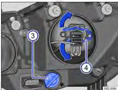
Fig. 174 No compartimento do motor: vista traseira do farol dianteiro direito sem cobertura de borracha: 3 indicadores de direção e 4 farol baixo.
