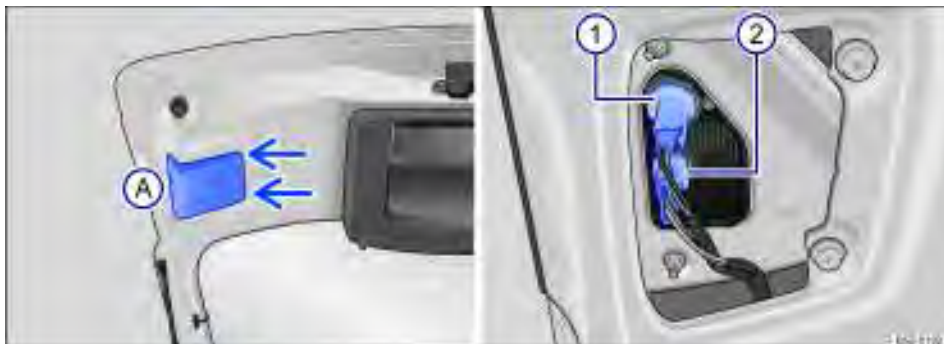
Fig. 179 Lanterna traseira: (A) desinstalar a cobertura e (1) e (2) desinstalar a lâmpada
