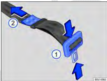
Fig. 53 Ajustar o cadarço do cinto de segurança subabdominal.
