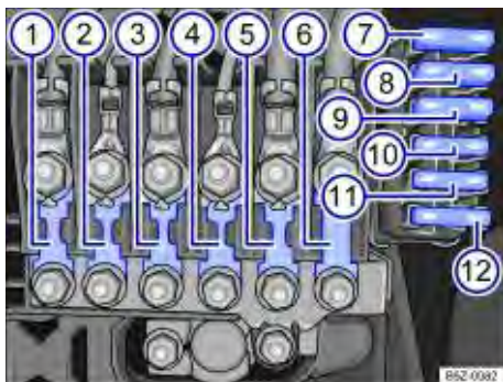
Fig. 172 Caixa de fusíveis.
