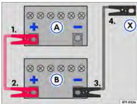
Fig. 184 Esquema para a conexão dos cabos auxiliares de partida: bateria do veículo descarregada e bateria do veículo fornecedora de corrente .
