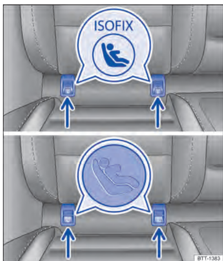
Fig. 3 No banco do veículo: variantes de identificação dos pontos de ancoragem ISOFIX para cadeiras de criança.
