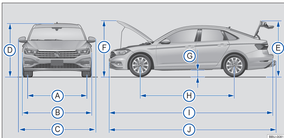
Fig. 13 Dimensões.
