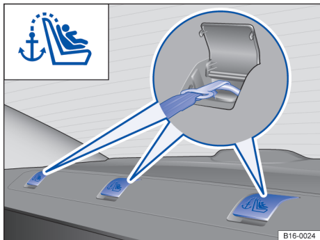
Fig. 5 Olhal de retenção na superfície atrás do encosto do banco traseiro.
