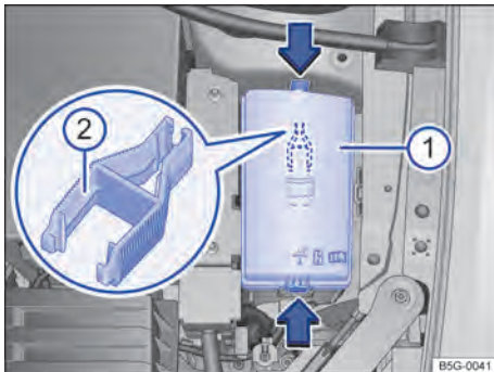
Fig. 150 No compartimento do motor: locais de instalação dos fusíveis.
