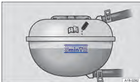
Fig. 167 No compartimento do motor: marcações no reservatório de expansão do líquido de arrefecimento (representação esquemática).
