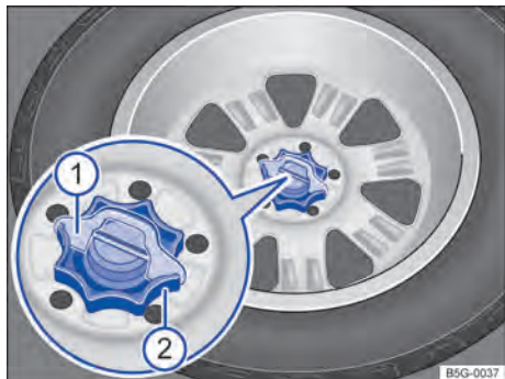
Fig. 185 No compartimento de bagagem: manipulô para fixaçã da roda sobressalente.
