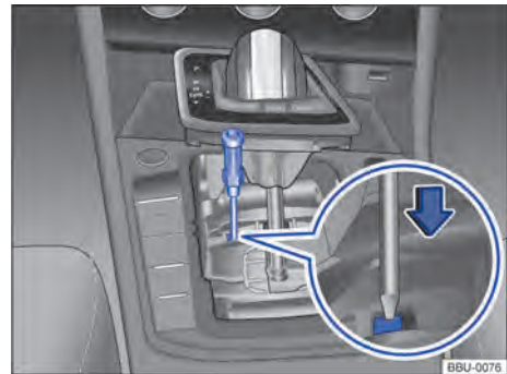
Fig. 110 Destravar emergencialmente o bloqueio da alavanca seletora.
