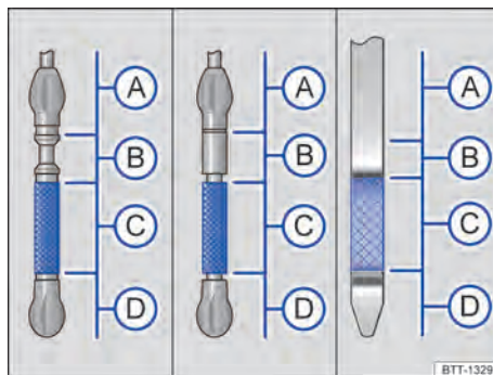
Fig. 165 Marcações do nível do óleo do motor na vareta de medição do óleo (variantes).
