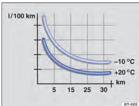
Fig. 99 Consumo de combustível em l/100 km em duas temperaturas ambiente diferentes.
