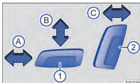
Fig. 73 Interruptor no banco dianteiro esquerdo: ajustar o banco dianteiro esquerdo na longitudinal, o assento do banco em altura e inclinação, bem como o encosto do banco dianteiro.
