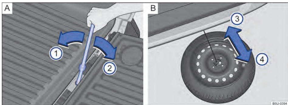
Fig. 165 A) No compartimento de carga: acesso a roda de emergência. B) Sob o veículo: roda de emergência totalmente no piso e retirada de baixo do veículo.
