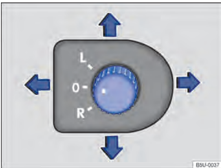
Fig. 72 Na porta do condutor: interruptor rotativo de ajuste dos espelhos retrovisores externos elétricos.
