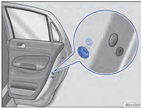
Fig. 37 Na porta traseira (lado direito): localização da trava de segurança para crianças.
