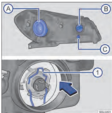
Fig. 108 No compartimento do motor: vista traseira do farol dianteiro com cobertura de borracha (lado esquerdo da ilustração) - A farol baixo / alto, B indicadores de direção e C luz de posição. Vista traseira do farol dianteiro sem a cobertura de borracha (lado direito da ilustração): 1 mola de travamento da lâmpada incandescente do farol baixo / alto.
