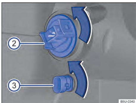
Fig. 109 No compartimento do motor: vista traseira do farol dianteiro 2 indicadores de direção e 3 luz de posição.
