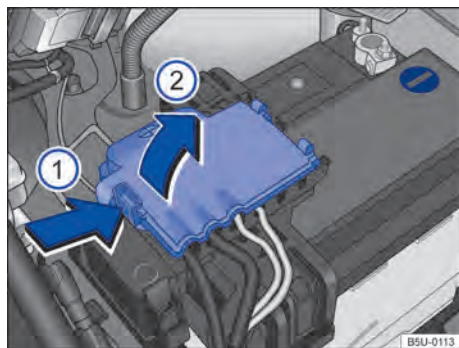
Fig. 122 Compartimento do motor: acesso ao terminal positivo da bateria.
