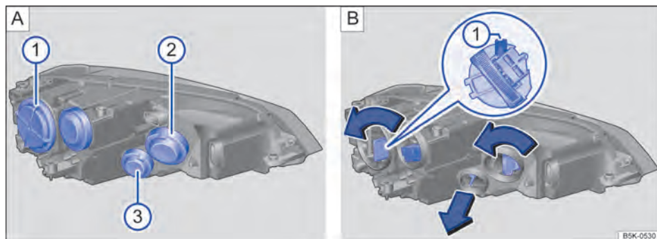
Fig. 197 No compartimento do motor: coberturas do farol dianteiro esquerdo. ① farol baixo, ② farol alto e luz de posição, bem como farol de rodagem diurna, ③ indicador de direção.
