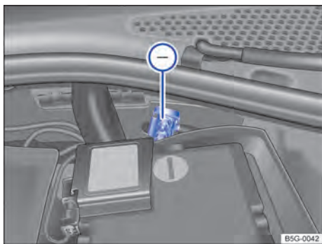
Fig. 216 No compartimento do motor: ponto de auxílio à partida (ponto de aterramento) ⓘ.
