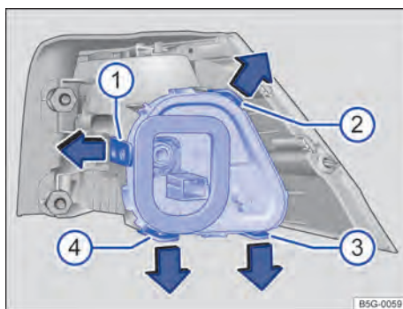
Fig. 203 Lanterna traseira da carroceria: desinstalar o suporte da lâmpada. Tiras de travamento ① a ④.
