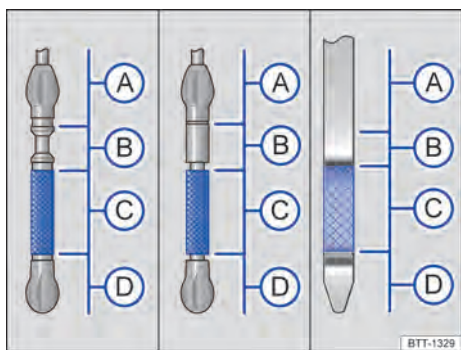
Fig. 226 Vareta de medição do óleo do motor com marcas de nível de óleo do motor.
