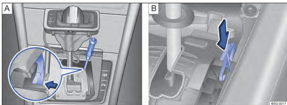
Fig. 127 Embaixa da cobertura do quadro da alavanca seletora: destravar o bloqueio da alavanca seletora emergencialmente, variante A e B .
