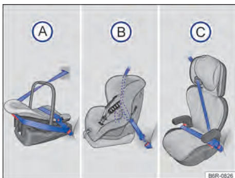
Fig. 46 As ilustrações (A), (B) e (C) mostram a fixação do sistema de retenção para crianças apenas com o cinto de segurança do veículo.
