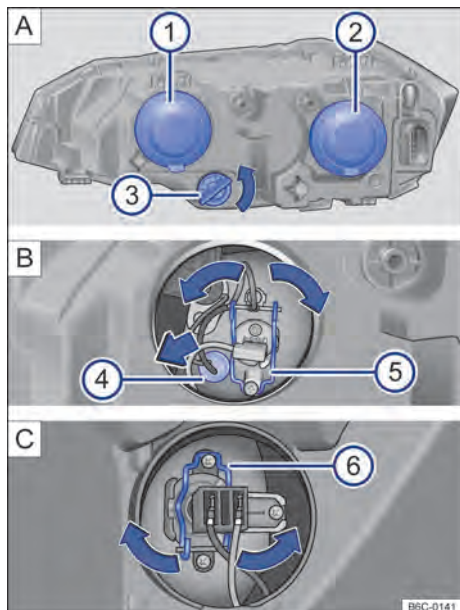
Fig. 136 No compartimento do motor: ① farol alto e luz de posição, ② farol baixo e ③ indicador de direção.
