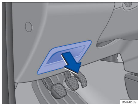
Fig. 152 No lado do condutor no painel de instrumentos: cobertura da caixa de fusíveis.
