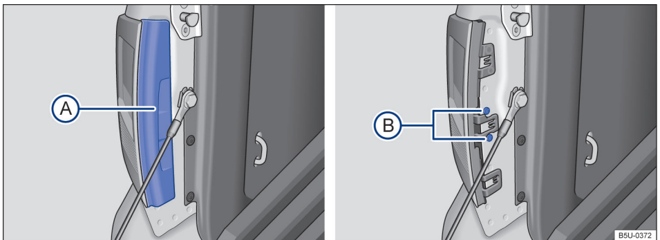
Fig. 146 No compartimento de carga: A desinstalar cobertura, B retirar os parafusos de fixação. ▶
