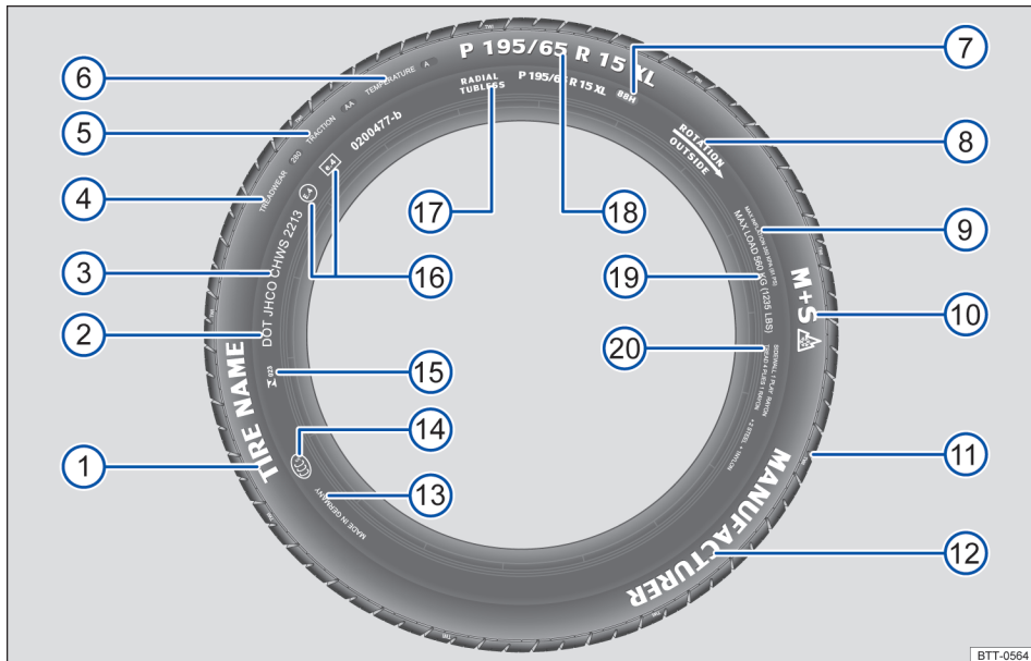
Fig. 176 Inscrição dos pneus internacional (exemplo).
