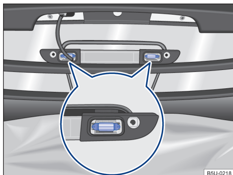
Fig. 151 Lanterna de freio elevada: remover a lâmpada incandescente da iluminação do compartimento de carga.
