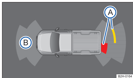
Fig. 101 Exibição do display do controle de distância de estacionamento (display colorido): A obstáculo reconhecido no segmento. B área examinada à frente do veículo.
