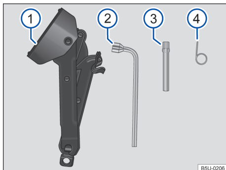
Fig. 137 Componentes das ferramentas de bordo.
