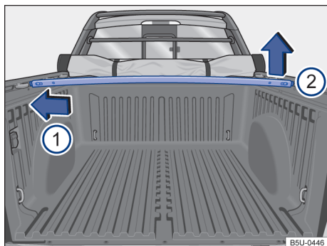
Fig. 59 Travessas no compartimento de carga: remover e instalar.
