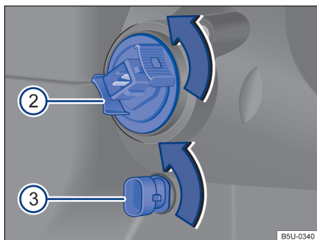
Fig. 140 No compartimento do motor: vista traseira do farol dianteiro 2 indicadores de direção e 3 luz de posição.
