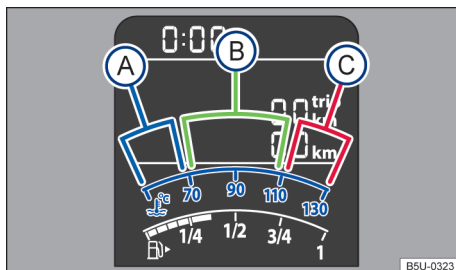
Fig. 16 Indicador de temperatura do líquido de arrefecimento do motor no instrumento combinado (variante 1): (A) área fria; (B) área normal; (C) área de alerta.
