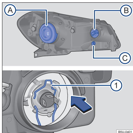
Fig. 139 No compartimento do motor: vista traseira do farol dianteiro com cobertura de borracha (lado esquerdo da ilustração) - A farol baixo / alto, B indicadores de direção e C luz de posição. Vista traseira do farol dianteiro sem a cobertura de borracha (lado direito da ilustração): 1 mola de travamento da lâmpada incandescente do farol baixo / alto.
