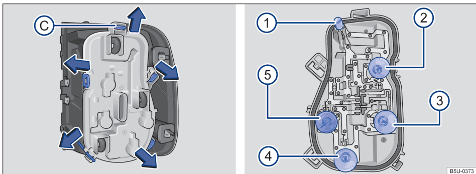
Fig. 147 Lanterna traseira: C desinstalar o suporte das lâmpadas e 1 , 2 , 3 , 4 e 5 desinstalar as lâmpadas.
