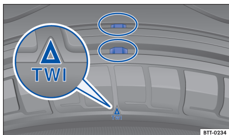
Fig. 173 Perfil do pneu: indicadores de desgaste.
