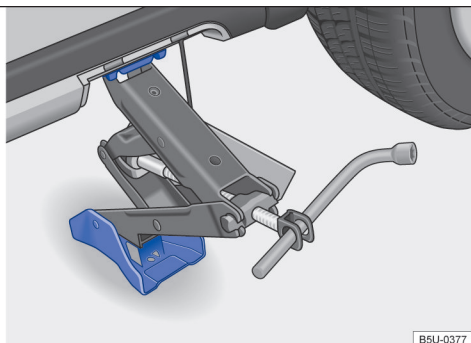
Fig. 181 Pontos de apoio do macaco e macaco posicionado no lado esquerdo traseiro do veículo - veículos com soleiras externas.
