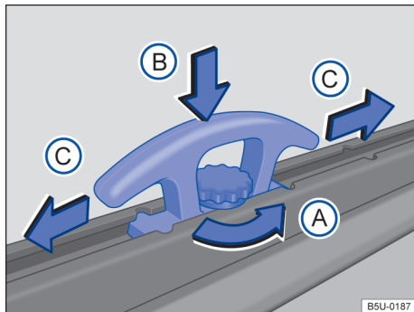
Fig. 127 No compartimento de carga: suporte deslizante para veículos sem capota marítima.
