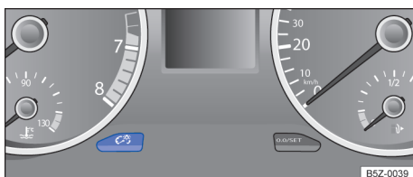
Fig. 73 No instrumento combinado: tecla de regulagem da iluminação dos instrumentos e dos interruptores.
