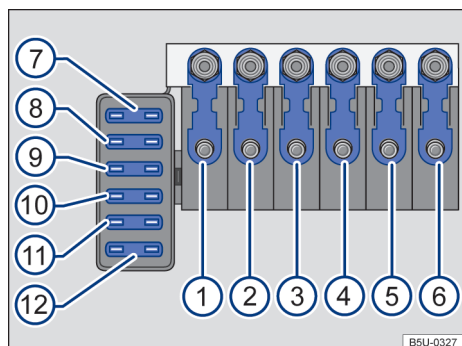
Fig. 155 Caixa de fusíveis.
