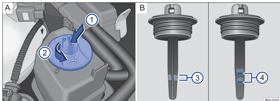
Fig. 93 No compartimento do motor (variante 1): A Reservatório do fluido da direção hidráulica. B Marcações para controle do nível do fluido da direção hidráulica.
