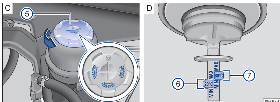
Fig. 94 No compartimento do motor (variante 2): C Reservatório do fluido da direção hidráulica. D Marcações para controle do nível do fluido da direção hidráulica.
