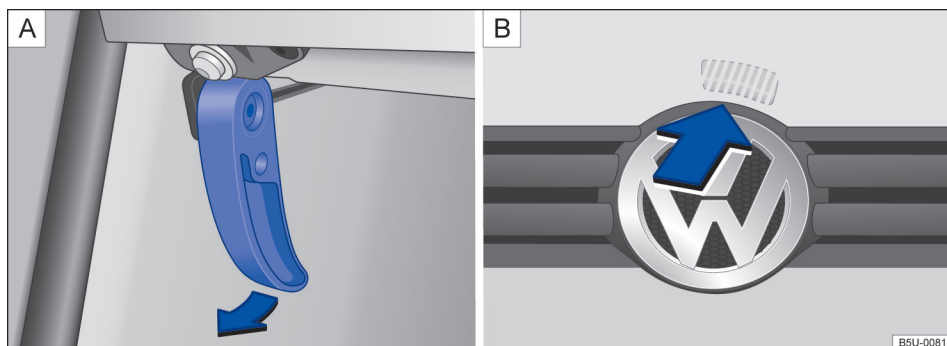
Fig. 160 A Alavanca de destravamento da tampa do compartimento do motor na área para os pés do lado do condutor. B Alavanca de destravamento na parte interna da tampa do compartimento do motor.
