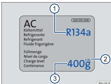
Fig. 190 Informações do ar-condicionado.
