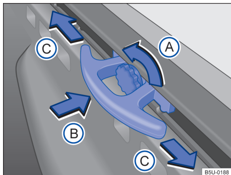
Fig. 128 No compartimento de carga: suporte deslizante para veículos com capota marítima.
