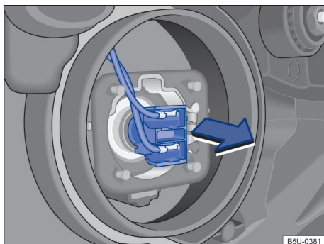
Fig. 142 Acesso à lâmpada incandescente do farol baixo.
