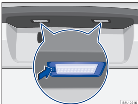
Fig. 148 No para-choque traseiro: remover a lanterna da placa de licença.
