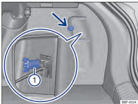
Fig. 141 No compartimento de bagagem: desinstalar cobertura e retirar o parafuso borboleta ① (lupa).
