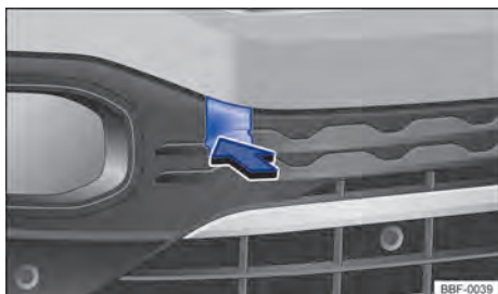
Fig. 152 No para-choque dianteiro à direita: soltar e remover a cobertura.
